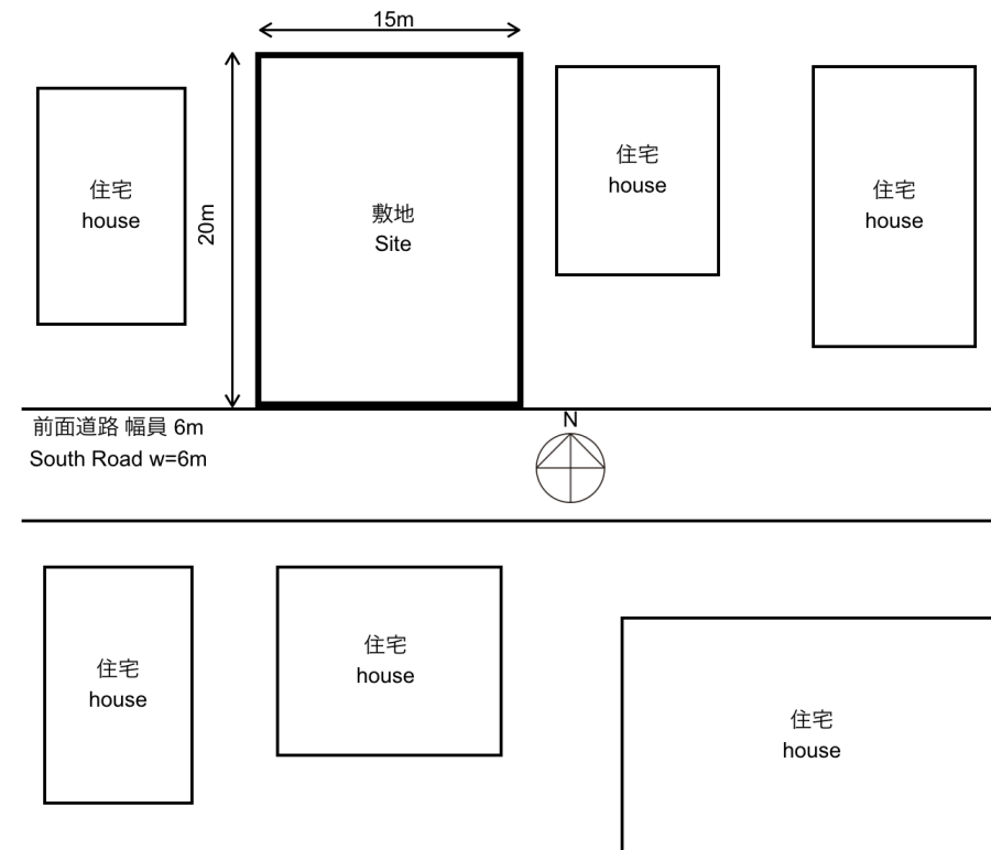
敷地図 Site plan
